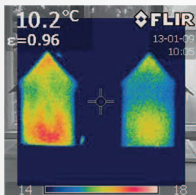
Rozdíl v propustnosti tepla po 5 minutách.
