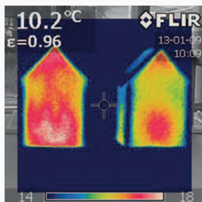
Rozdíl v propustnosti tepla po 10 minutách.
