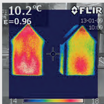
A makett falán átjutó hő képe 10 perc után.
