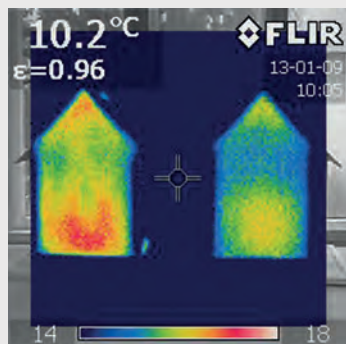
A makett falán átjutó hő képe 5 perc után.
